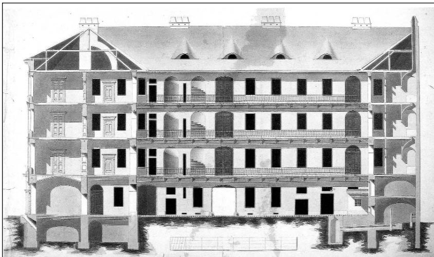
A Strohmayer-ház. Schmidt Antal tervrajza
